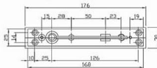
Bộ phận trên cánh cửa Top pivot (Door side)
