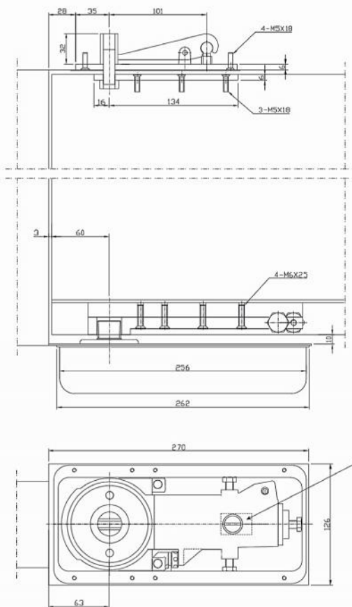
Bộ phận trên khung cửa Top pivot (Top jamb side)
