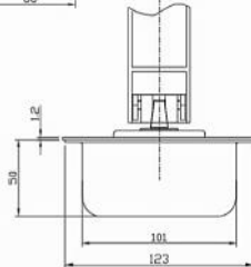
Ốc gia cố, mã số độc quyền Trung Quốc (China patent No): ZL 97 2 34782. 8
