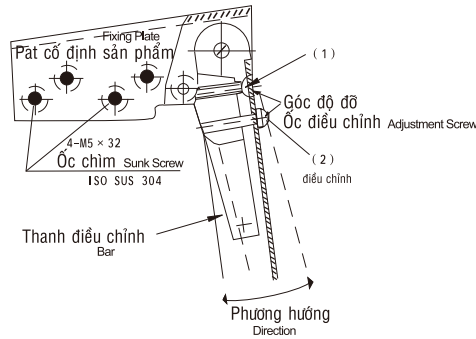
Bản vẽ canh chỉnh
