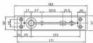
Bộ phận trên cánh cửa Top pivot (Door side)
