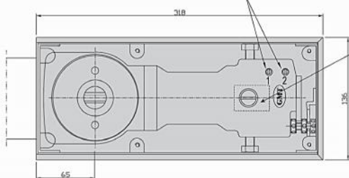
Ốc điều chỉnh tốc độ đóng Closing Speed Adjustment Valve
